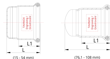
Technický náčres
