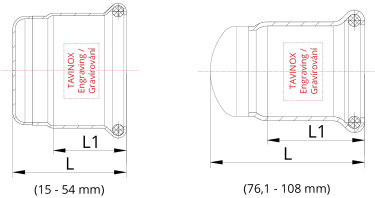
Technický nákres
