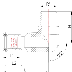
Technische Zeichnung
