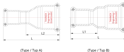
Technische Zeichnung
