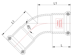
Technische Zeichnung
