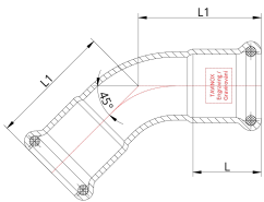
Technische Zeichnung
