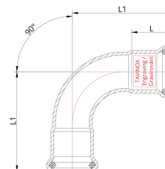
Technische Zeichnung
