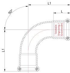
Technische Zeichnung
