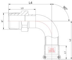
Technische Zeichnung
