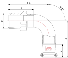
Technische Zeichnung
