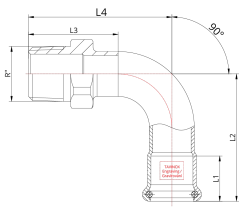
Technische Zeichnung
