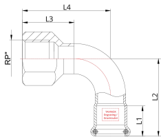
Technische Zeichnung
