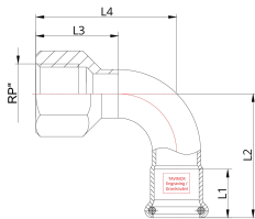
Technische Zeichnung
