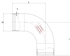
Technische Zeichnung
