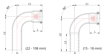
Technische Zeichnung
