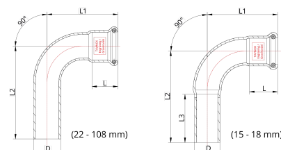
Technische Zeichnung
