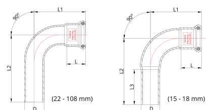
Technische Zeichnung
