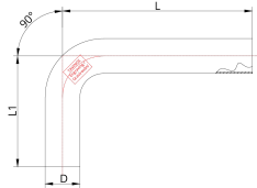
Technische Zeichnung
