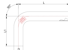
Technische Zeichnung
