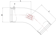
Technische Zeichnung
