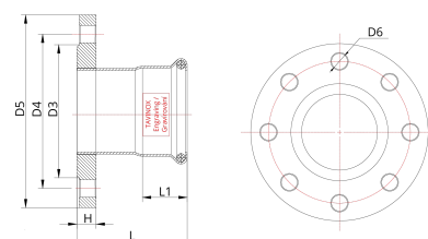
Technische Zeichnung
