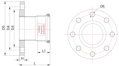
Technische Zeichnung
