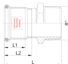
Technische Zeichnung
