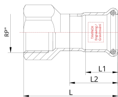
Technische Zeichnung
