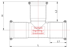
Technische Zeichnung
