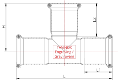
Technische Zeichnung
