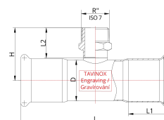
Technische Zeichnung
