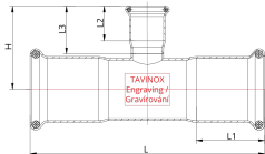
Technische Zeichnung
