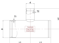
Technische Zeichnung
