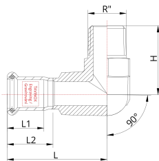
Технічне креслення
