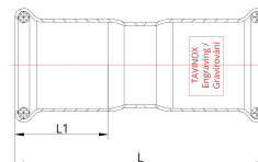
Технічне креслення
