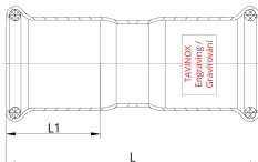
Технічне креслення
