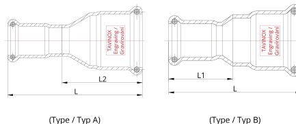
Технічне креслення
