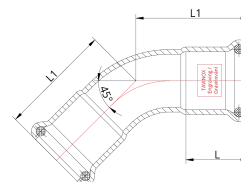
Технічне креслення
