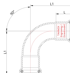
Технічне креслення
