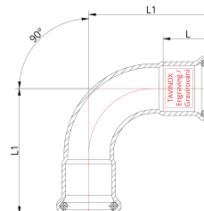
Технічне креслення
