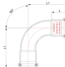
Технічне креслення
