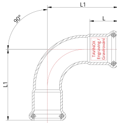
Технічне креслення
