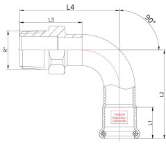
Технічне креслення
