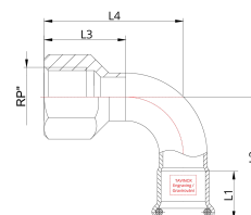
Технічне креслення
