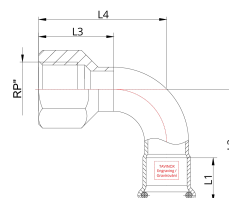
Технічне креслення
