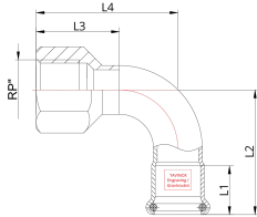
Технічне креслення
