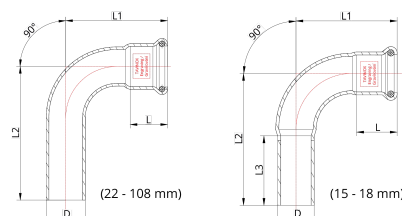
Технічне креслення
