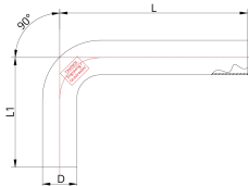
Технічне креслення
