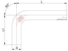
Технічне креслення
