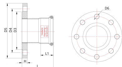
Технічне креслення
