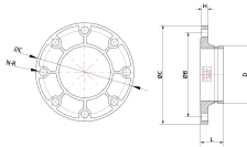
Технічне креслення
