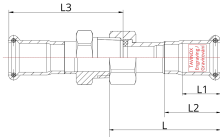
Технічне креслення
