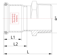
Технічне креслення
