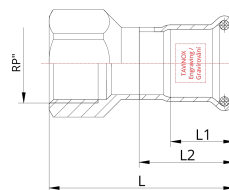
Технічне креслення
